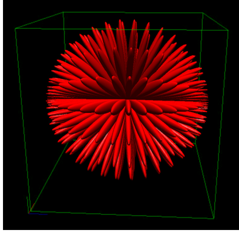
FIG. 9. \sin(9\theta) \cdot \sin(18\phi) - R = 0
