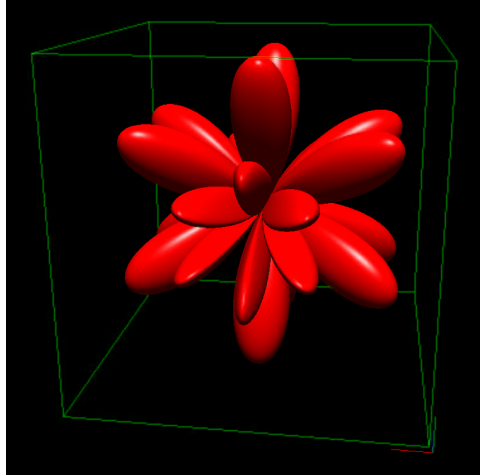
FIG. 14. \sin(3\theta) \cdot \sin(4\phi) - R = 0
